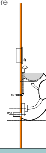
Robinet indépendant
