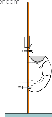
Robinet indépendant
